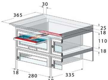
mod. orizzontale profondo
