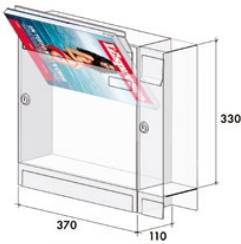
mod. EURO 37F
