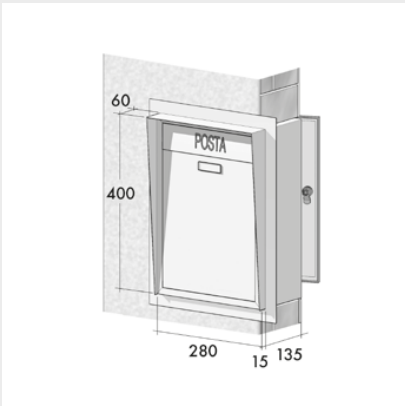
VERSIONE 2 Da incasso a due frontali
