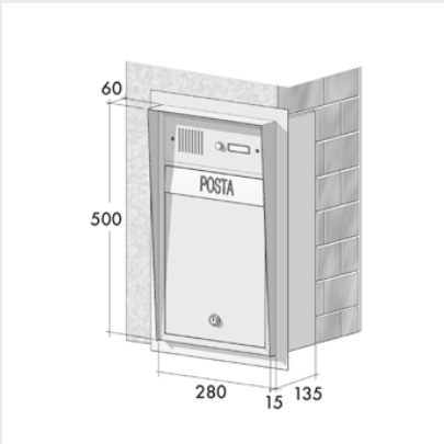
VERSIONE 5 Da incasso con citofono
