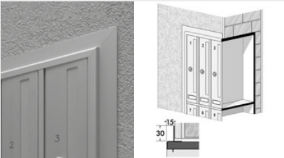
Incasso a muro con profilo coprifuga piatto h. cm. 3.
