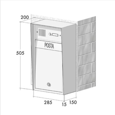
VERSIONE 7 Da appendere con citofono
