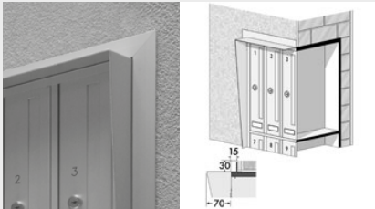
Incasso a muro con profilo coprifuga piatto h. cm. 3 più tetto parapioggia da cm 6/8/10.
