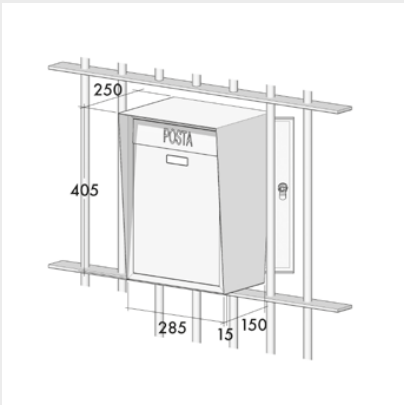
VERSIONE 4 Passante a due frontali per cancello
