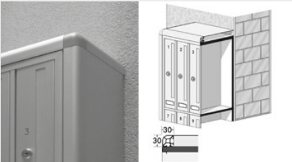
Inserimento in cassetto d'alluminio modulare a spigoli tondi, installazione a parete, in recinzione, autoportante con piantane.
