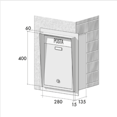
VERSIONE 1 Da incasso
