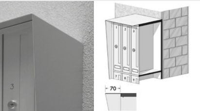
Tetto e schienale in alluminio, installazione a parete, in recinzioni, autoportante con piantane.
