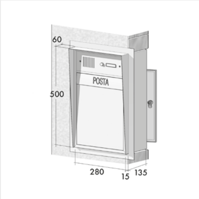
VERSIONE 6 Da incasso con citofono a due frontali
